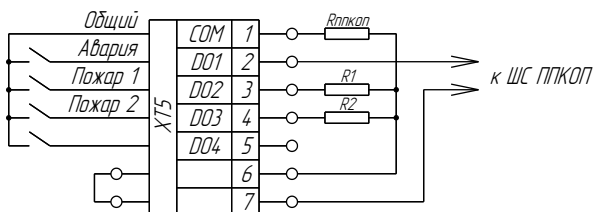
Схема подключения выходов клеммника XT5 в шлейф пожарной сигнализации
